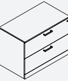
FDR400 FDR400-65: W 90 x D 51.6 x H 65
