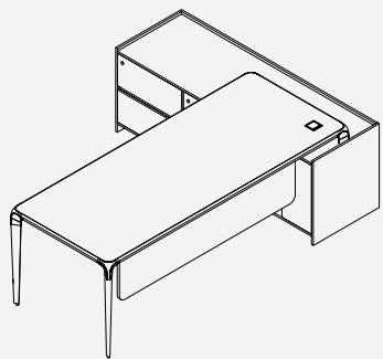
CM300 CM300-180: W 180 x D 90 x H 76 (Total Dim: 205x180x76) CM300-200: W 200 x D 90 x H 76 (Total Dim: 225x180x76) CM300-220: W 220 x D 90 x H 76 (Total Dim: 245x180x76) Sideboard: W 180 x D 60 x H 66
