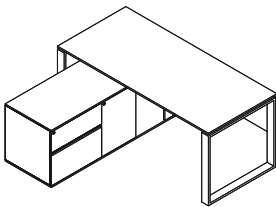
BM 300 BM200-180 : W 180 x D 80 x H 76 BM200-200 : W 200 x D 80 x H 76 BM200-220 : W 220 x D 85 x H 76 Sideboard : W 150 x D 55 x H 60
