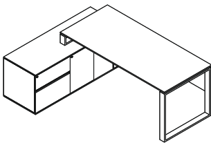
BM 200 BM200-180 : W 180 x D 80 x H 76 BM200-200 : W 200 x D 80 x H 76 BM200-220 : W 220 x D 85 x H 76 Sideboard : W 150 x D 55 x H 60
