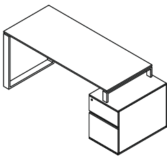
BD 200 BD200-120 : W 120 x D 70 x H 76 BD200-140 : W 140 x D 70 x H 76 BD200-160 : W 160 x D 70 x H 76 Sideboard : W 750 x D 45 x H 60
