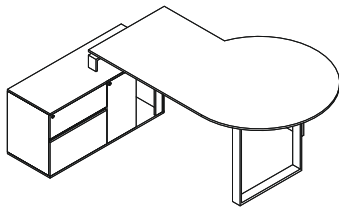
BM 100 BM100-180 : W 180 x D 120 x H 76 BM100-200 : W 200 x D 120 x H 76 Sideboard : W 120 x D 45 x H 60
