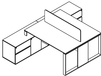
BW 200 BW200-120 : W 120 x D 150 x H 76 BW200-140 : W 140 x D 150 x H 76 BW200-160 : W 160 x D 150x H 76 Sideboard : W 260 x D 50 x H 70
