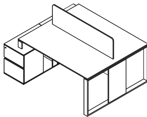
BW 100 BW200-120 : W 120 x D 140 x H 76 BW200-140 : W 140 x D 140 x H 76 BW200-160 : W 160 x D 140x H 76 Sideboard : W 160 x D 45 x H 60
