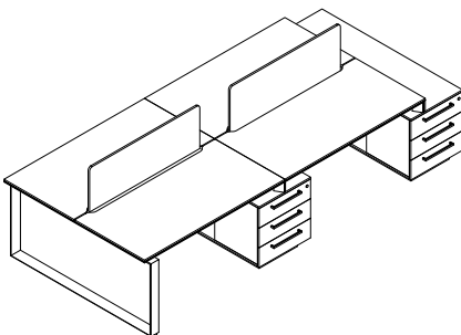
TW300 TW300-240 : W 240 x D 150 x H 76 TW300-280 : W 280 x D 150 x H 76 TW300-300 : W 300 x D 150 x H 76 TW300-320 : W 320 x D 150 x H 76 TW300-360 : W 360 x D 150 x H 76 Sideboard : W 150 x D 55 x H 64.1
