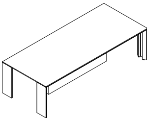
ECO200 ECO200-120 : W 120 x D 120 x H 76 ECO200-180 : W 180 x D 120 x H 76 ECO200-240 : W 240 x D 120 x H 76 ECO200-300 : W 300 x D 120 x H 76
