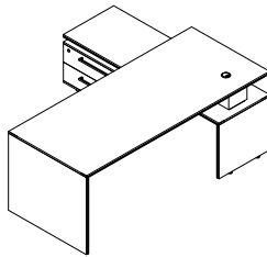
EM300 EM300-180 : W 180 x D 80 x H 76 EM300-200 : W 200 x D 80 x H 76 EM300-220 : W 220 x D 85 x H 76 EM300-240 : W 240 x D 85 x H 76 Pedestal : W 170 x D 55 x H 58.8
