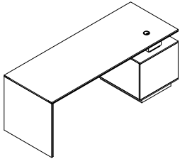
ED300 ED300-140 : W 140 x D 75 x H 76 ED300-160 : W 160 x D 75 x H 76 ED300-180 : W 180 x D 75 x H 76 ED300-200 : W 200 x D 75 x H 76 Pedestal : W 60 x D 75 x H 60
