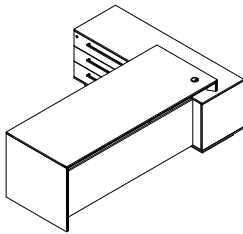
EM100 EM100-180 : W 180 x D 80 x H 76 EM100-200 : W 200 x D 80 x H 76 EM100-220 : W 220 x D 85 x H 76 EM100-240 : W 240 x D 85 x H 76 Sideboard : W 170 x D 55 x H 64.1
