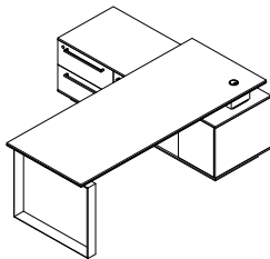
PM100 PM100-180 : W 180 x D 80 x H 76 PM100-200 : W 200 x D 80 x H 76 PM100-220 : W 220 x D 85 x H 76 PM100-240 : W 240 x D 85 x H 76 Pedestal : W 170 x D 55 x H 58.8
