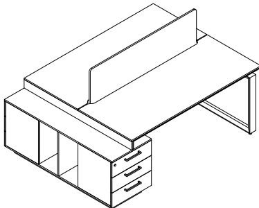
TW400 TW400-120 : W 120 x D 150 x H 76 TW400-140 : W 140 x D 150 x H 76 TW400-160 : W 160 x D 150 x H 76 TW400-180 : W 180 x D 150 x H 76 TW400-200 : W 200 x D 150 x H 76 Sideboard : W 150 x D 55 x H 64.1
