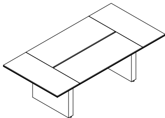
ECO100 ECO100-200 : W 200 x D 100 x H 76 ECO100-260 : W 260 x D 110 x H 76 ECO100-330 : W 330 x D 120 x H 76 ECO100-420 : W 420 x D 140 x H 76 ECO100-480 : W 480 x D 140 x H 76
