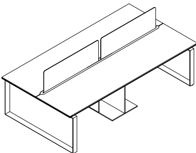
TW600 TW600-240 : W 240 x D 150 x H 76 TW600-280 : W 280 x D 150 x H 76 TW600-300 : W 300 x D 150 x H 76 TW600-320 : W 320 x D 150 x H 76 TW600-360 : W 360 x D 150 x H 76
