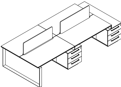
TW300 TW300-240 : W 240 x D 150 x H 76 TW300-280 : W 280 x D 150 x H 76 TW300-300 : W 300 x D 150 x H 76 TW300-320 : W 320 x D 150 x H 76 TW300-360 : W 360 x D 150 x H 76 Sideboard : W 150 x D 55 x H 64.1
