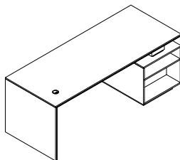
ED400 ED400-140 : W 140 x D 75 x H 76 ED400-160 : W 160 x D 75 x H 76 ED400-180 : W 180 x D 75 x H 76 ED400-200 : W 200 x D 75 x H 76 Pedestal : W 60 x D 75 x H 60
