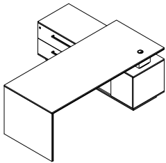
EM200 EM200-180 : W 180 x D 80 x H 76 EM200-200 : W 200 x D 80 x H 76 EM200-220 : W 220 x D 85 x H 76 EM200-240 : W 240 x D 85 x H 76 Pedestal : W 170 x D 55 x H 58.8
