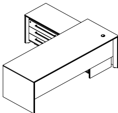
EM400 EM400-180 : W 180 x D 80 x H 76 EM400-200 : W 200 x D 80 x H 76 EM400-220 : W 220 x D 85 x H 76 EM400-240 : W 240 x D 85 x H 76 Sideboard : W 170 x D 55 x H 67
