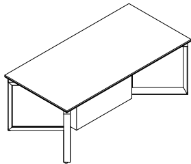
TCO100 TCO100-160 : W 160 x D 120 x H 76 TCO100-220 : W 220 x D 120 x H 76 TCO100-280 : W 280 x D 120 x H 76
