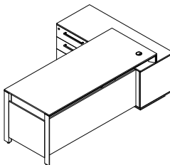
EM500 EM500-180 : W 180 x D 80 x H 76 EM500-200 : W 200 x D 80 x H 76 EM500-220 : W 220 x D 85 x H 76 EM500-240 : W 240 x D 85 x H 76 Sideboard : W 140 x D 55 x H 64.1
