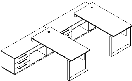
TW100 TW100-120 : W 120 x D 75 x H 76 TW100-140 : W 140 x D 75 x H 76 TW100-160 : W 160 x D 75 x H 76 TW100-180 : W 180 x D 75 x H 76 TW100-200 : W 200 x D 75 x H 76 Sideboard : W 170 x D 55 x H 64.1
