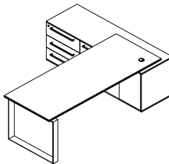
PM200 PM200-180 : W 180 x D 80 x H 76 PM200-200 : W 200 x D 80 x H 76 PM200-220 : W 220 x D 85 x H 76 PM200-240 : W 240 x D 85 x H 76 Sideboard : W 170 x D 55 x H 69
