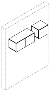
FL300 FL300-45 : W 45 x D 36.6 x H 37.5 FL300-90 : W 90 x D 36.6 x H 37.5
