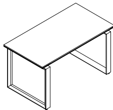
PD100 PD100-140 : W 140 x D 75 x H 76 PD100-160 : W 160 x D 75 x H 76 PD100-180 : W 180 x D 75 x H 76 PD100-200 : W 200 x D 75 x H 76
