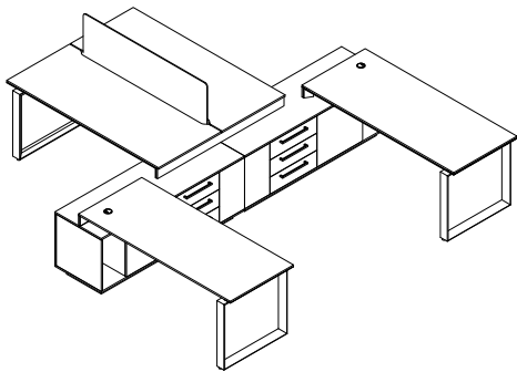
TW200 TW200-120 : W 120 x D 75 x H 76 TW200-140 : W 140 x D 75 x H 76 TW200-160 : W 160 x D 75 x H 76 TW200-180 : W 180 x D 75 x H 76 TW200-200 : W 200 x D 75 x H 76 Sideboard : W 170 x D 55 x H 64.1
