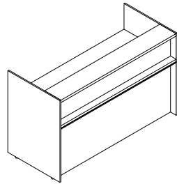
ER200 ER200-180 : W 180 x D 80 x H 110 ER200-200 : W 200 x D 80 x H 110 ER200-220 : W 220 x D 80 x H 110
