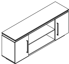
ECR100 ECR100-180 : W 180 x D 45 x H 76 ECR100-200 : W 200 x D 45 x H 76 ECR100-220 : W 220 x D 45 x H 76
