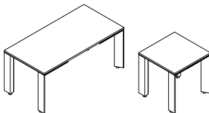
TA100 TA100-45 : W 45 x D 45 x H 45 TA100-90 : W 90 x D 90 x H 45 TA100-100 : W 100 x D 50 x H 45 TA100-120 : W 120 x D 120 x H 45
