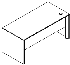
ED100 ED100-140 : W 140 x D 75 x H 76 ED100-160 : W 160 x D 75 x H 76 ED100-180 : W 180 x D 75 x H 76 ED100-200 : W 200 x D 75 x H 76
