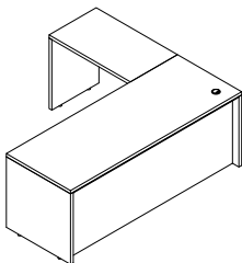
TD200 TD200-120 : W 120 x D 70 x H 76 TD200-140 : W 140 x D 75 x H 76 TD200-160 : W 160 x D 75 x H 76 TD200-180 : W 180 x D 75 x H 76 Sideboard : W 100 x D 55 x H 76
