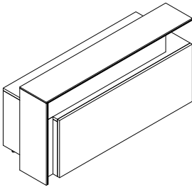
ER300 ER300-180 : W 180 x D 80 x H 110 ER300-200 : W 200 x D 80 x H 110 ER300-220 : W 220 x D 80 x H 110
