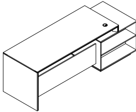
ED200 ED200-140 : W 140 x D 75 x H 76 ED200-160 : W 160 x D 75 x H 76 ED200-180 : W 180 x D 75 x H 76 ED200-200 : W 200 x D 75 x H 76 Sideboard : W 80 x D 75 x H 64.1
