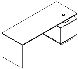
ED300 ED300-140 : W 140 x D 75 x H 76 ED300-160 : W 160 x D 75 x H 76 ED300-180 : W 180 x D 75 x H 76 ED300-200 : W 200 x D 75 x H 76 Pedestal : W 60 x D 75 x H 60
