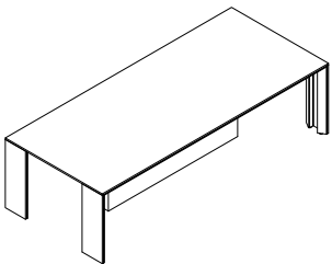
ECO200 ECO200-120 : W 120 x D 120 x H 76 ECO200-180 : W 180 x D 120 x H 76 ECO200-240 : W 240 x D 120 x H 76 ECO200-300 : W 300 x D 120 x H 76
