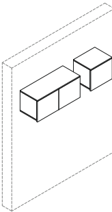
FL300 FL300-45 : W 45 x D 36.6 x H 37.5 FL300-90 : W 90 x D 36.6 x H 37.5
