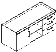
FWH400 FWH400-60 : W 135 x D 51.6 x H 60
